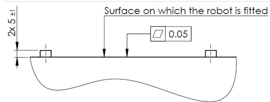
1.2: 로봇 베이스용 장착 플레이트
